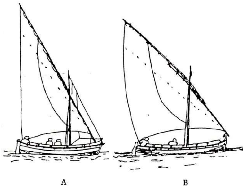
Fig. 1 Voile. La voile est de deux formes... ou pointue (espigado), fig. A, ou se rapprochant de la forme catalane (roundo), fig. B
