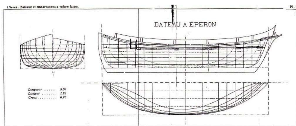
Fig. 2 Bateau à éperon
